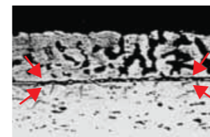
Penampang melintang mikroskopis AZ100 100 gram lapisan paduan Aluminium-Zinc setiap m 2
