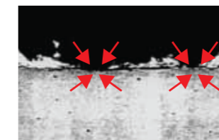
Penampang melintang mikroskopis Baja Galvanis Z120 120 gram lapisan Zinc setiap m 2
