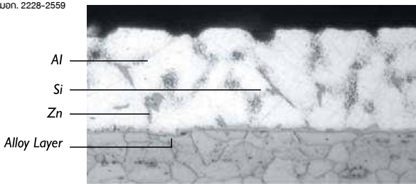
ภาพตัดโครงสร้างทางจุลภาคของเหล็กเคลือบโลหะสังกะสี-อะลูมิเนียม Microstructure Cross Section of Zincalume® steel
