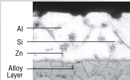
ภาพตัดโครงสร้างทางจุลภาคของเหล็กเคลือบโลหะซิงคาลูม Microstructure cross section of ZINCALUME® steel
